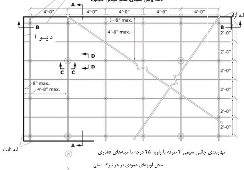
شکل پ ۶-۳۳- پلان مهاربندی عرضی برای شبکه سقف سنگین معلق (جزئیات مقاطع در شکل پ ۶-۲۹ ارائه شده است)
